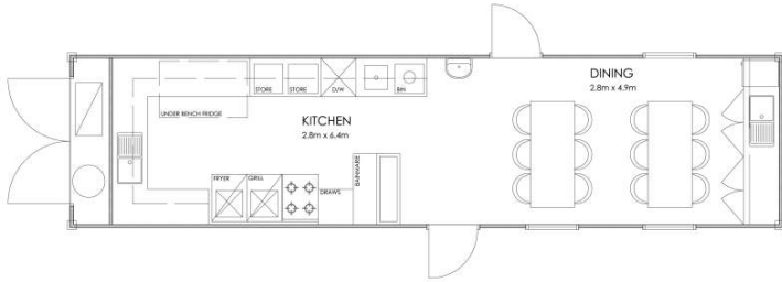
SERVERY MODULE (40FMOSERVE01) 12192 OR 6096 x 3000 x 2896 at 2500kg - 6000kg approx
